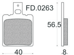
98.1061 Sinter Fr. 27.60
